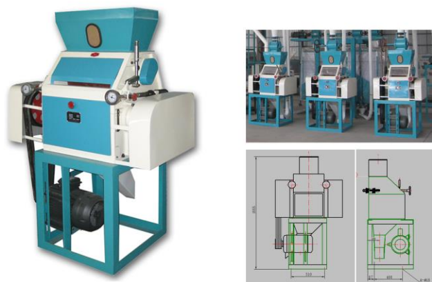
S-Roller Mill
